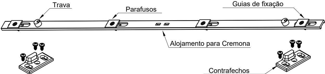
PERSPECTIVA: (Escala 1:4)
