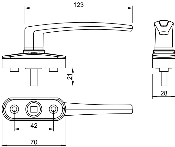
DIMENSÕES: (Escala 1:2)
