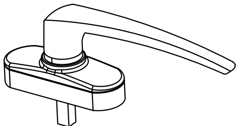
PERSPECTIVA: (Escala 1:2)
